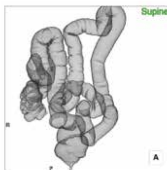
図2.仮想注腸像
